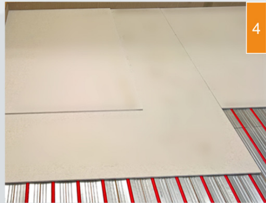
(4) De Fermacellplaten worden gelegd.
