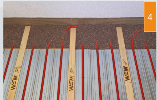
(4) De delen rond de bochten worden met isolatiekorrels gevuld.
