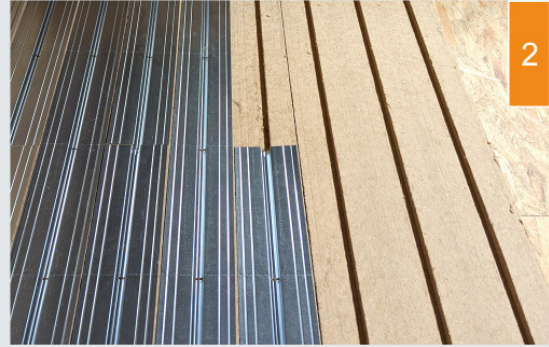
(2) Warmtegeleidende metaalplaten worden in de vloerplaten gelegd.
